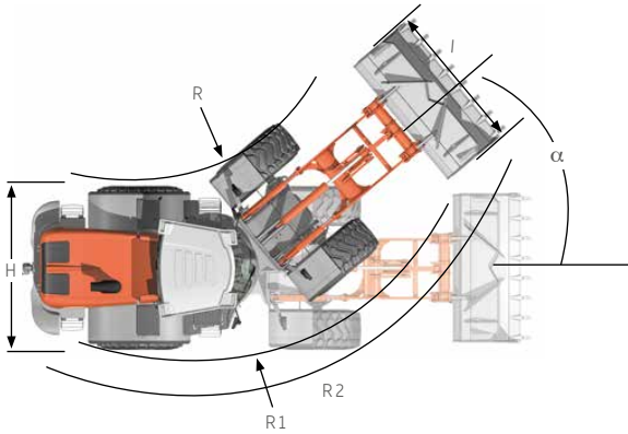
Avec attache rapide et godet standard
