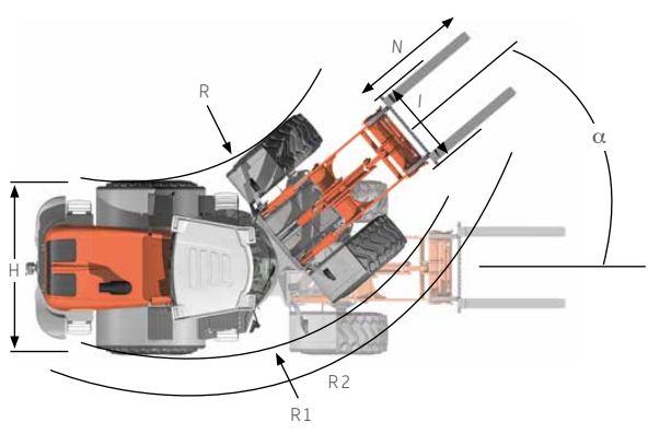
Avec attache rapide fourche à palette 1 400 mm
